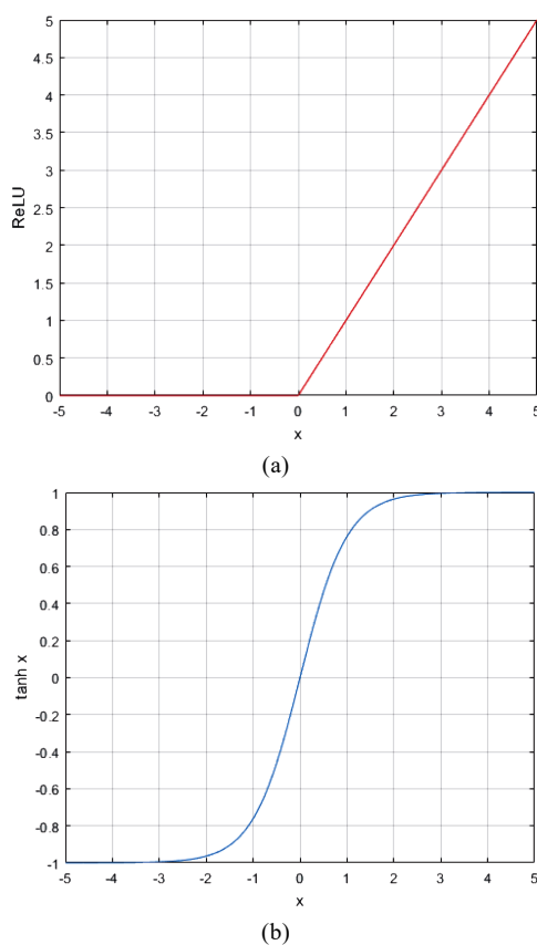
图4 ReLU 和 tanh 函数图像 Fig.4 ReLU and tanh function images
