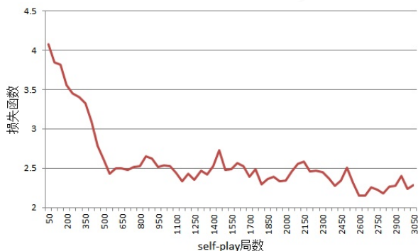
图 6 损失函数 Fig.6 Loss function
